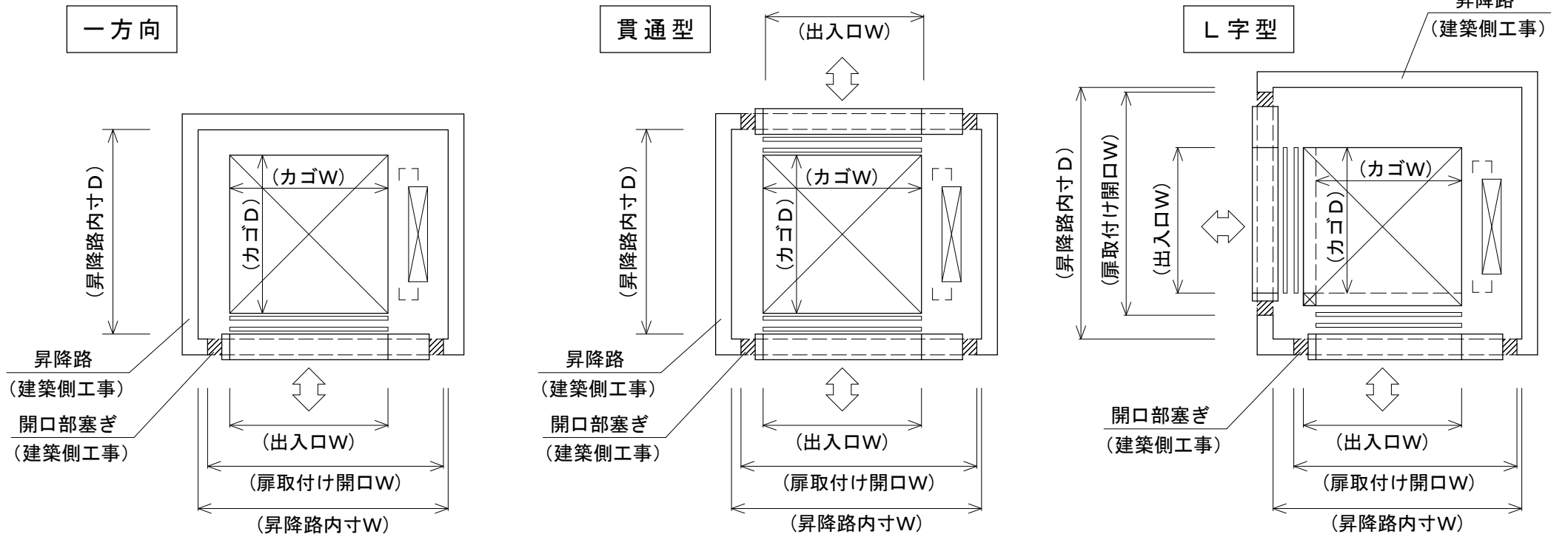
<平面図>
